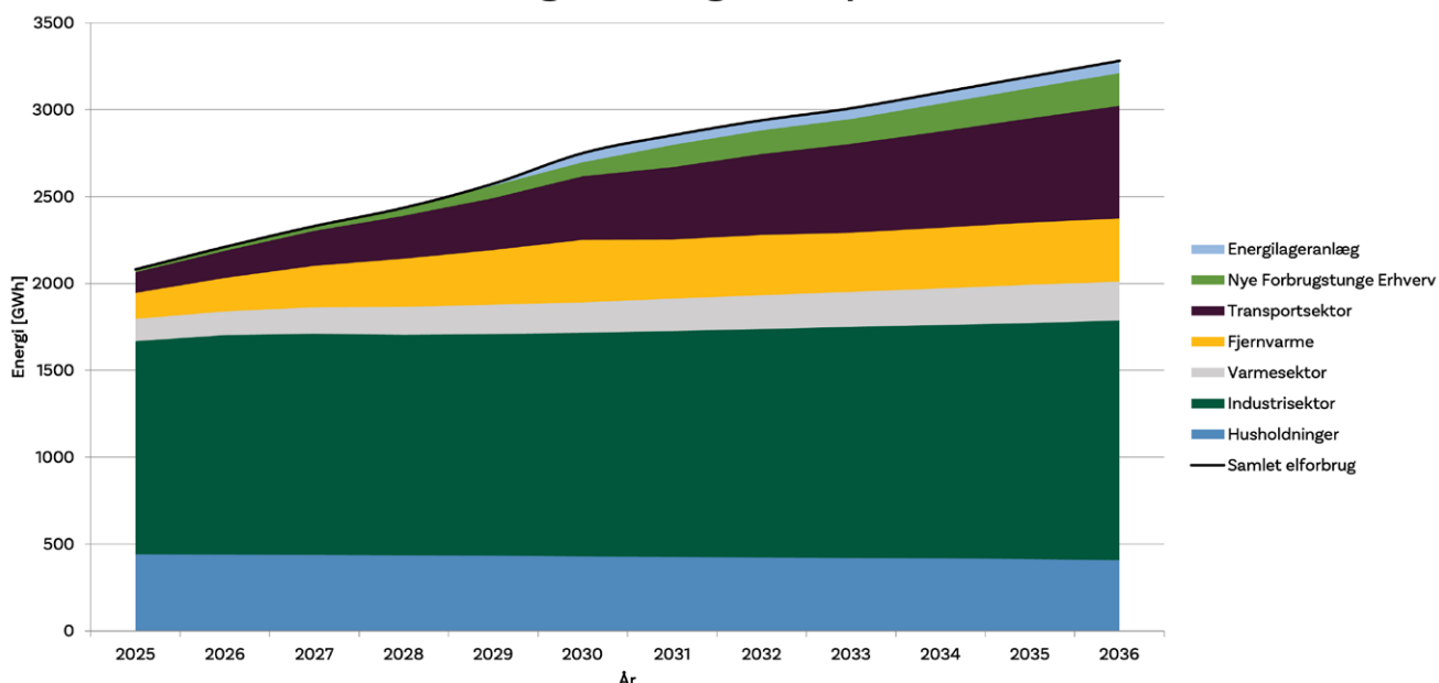
Figur 3: Udvikling i forventet elforbrug 2025-2036 fordelt på sektorer.
