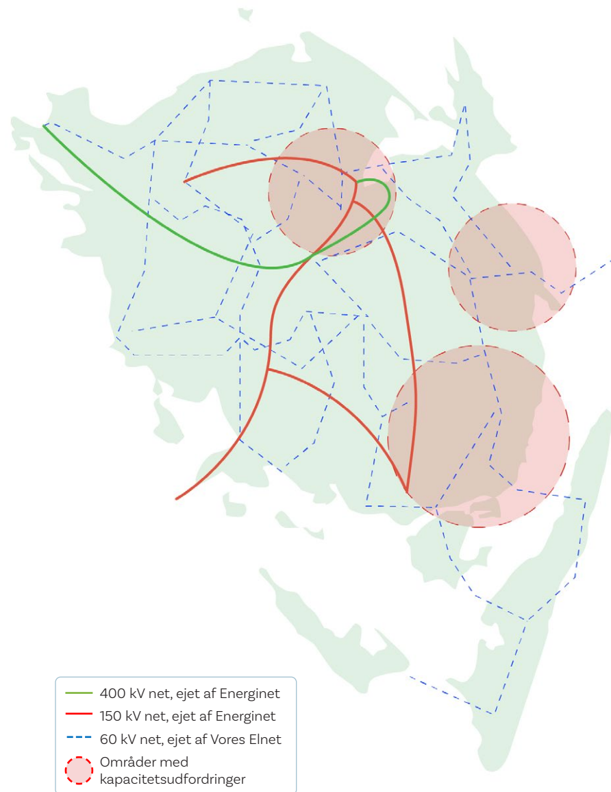
Figur 5: Illustration over elnettet på Fyn og Øerne.
