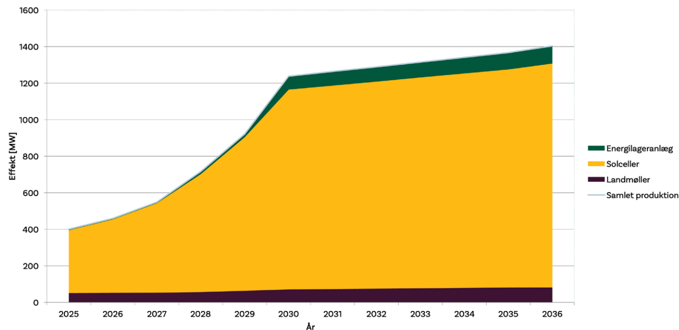
Udvikling i elproduktion fordelt på produktionskilder
