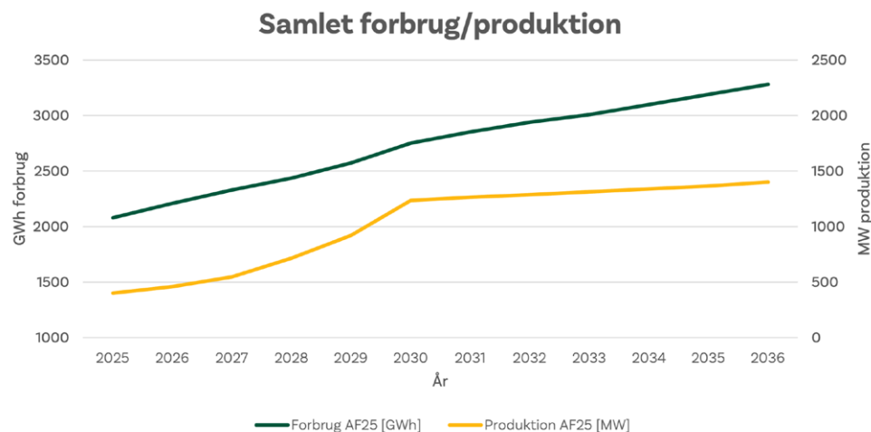
Figur 2: Udvikling i samlet elforbrug og elproduktion på Fyn og Øerne i 2025-2036.
